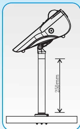
窄擠桌面(VESA方式)
